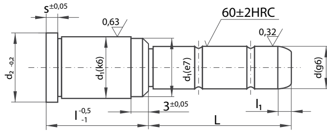
Mat.: 1.7131 Nawęglany / Carbonized
